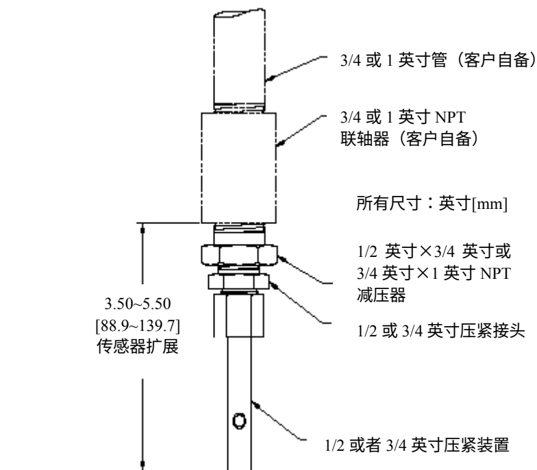
图 2-4 浸入式安装详图
